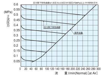
【ハイ・セレクト調整器 流量表】 GHN-4/GHSS-4
